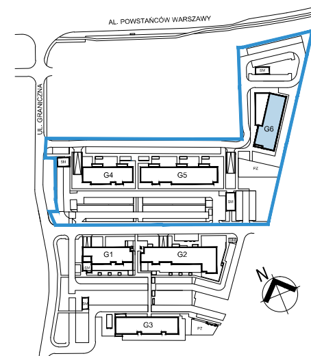
PLAN ZAGOSPODAROWANIA
